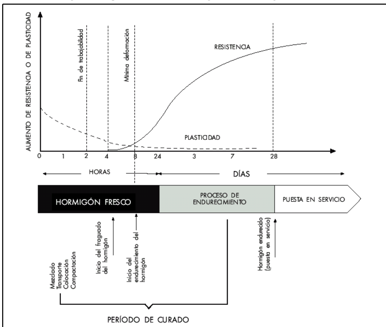
Figura 2.- Etapas de transición del hormigón fresco a hormigón endurecido.
