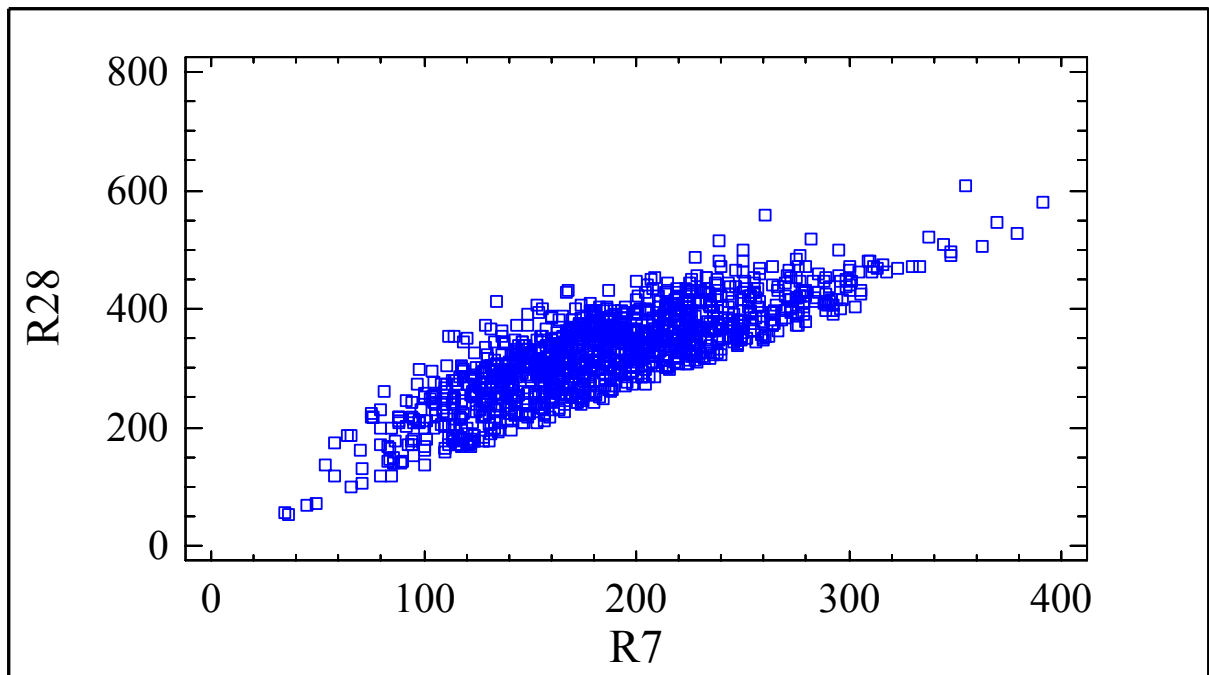
Gráfico 24.- Gráfico de Dispersión R_{28} v/s R_7 ( \text{Kg/cm}^2 )
