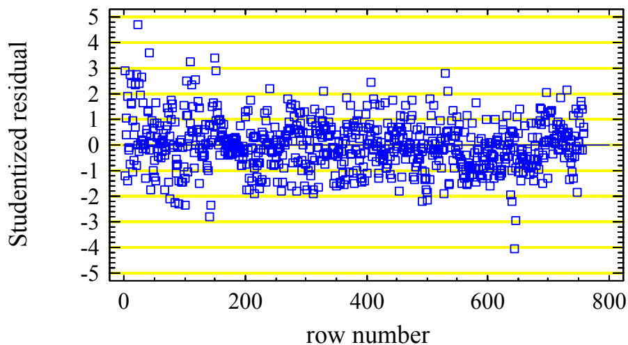
Gráfico 20.- Residual Plot
