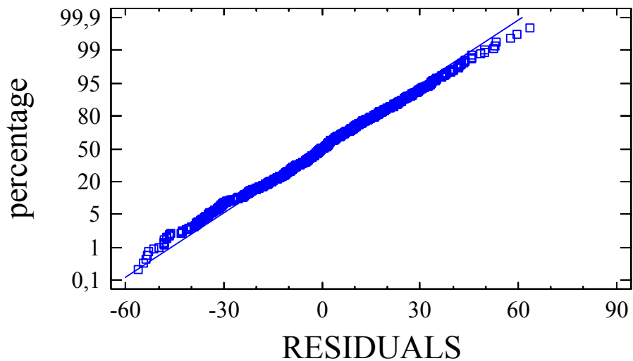
Gráfico 23.- Normal Probability Plot
