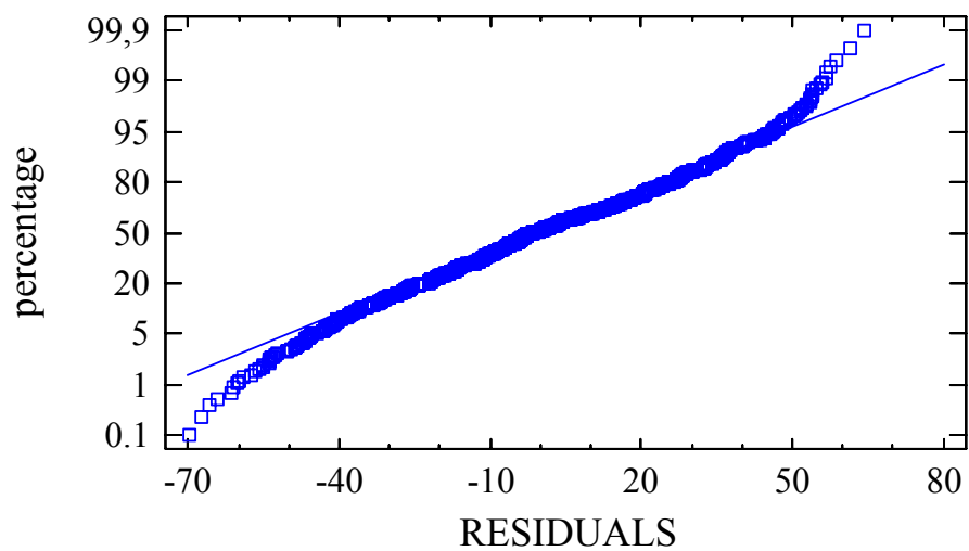
Gráfico 33.- Normal Probability Plot
