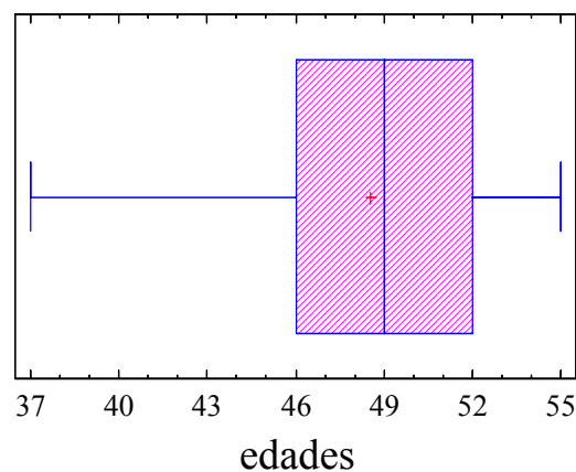
Gráfico 2.- Box-and-Whisker Plot
