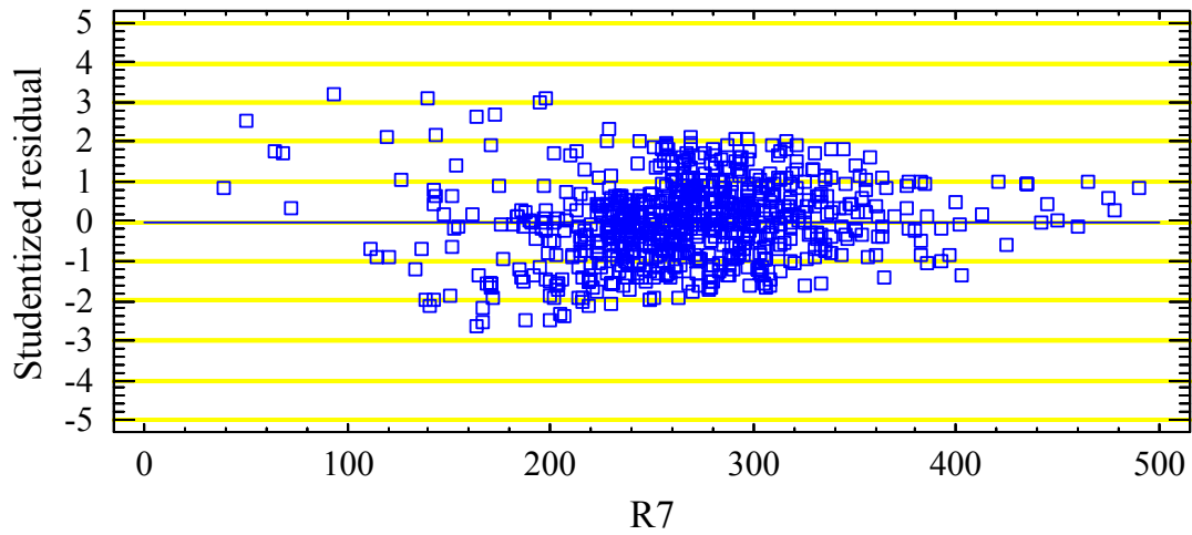
Gráfico 21.- Residual Plot
