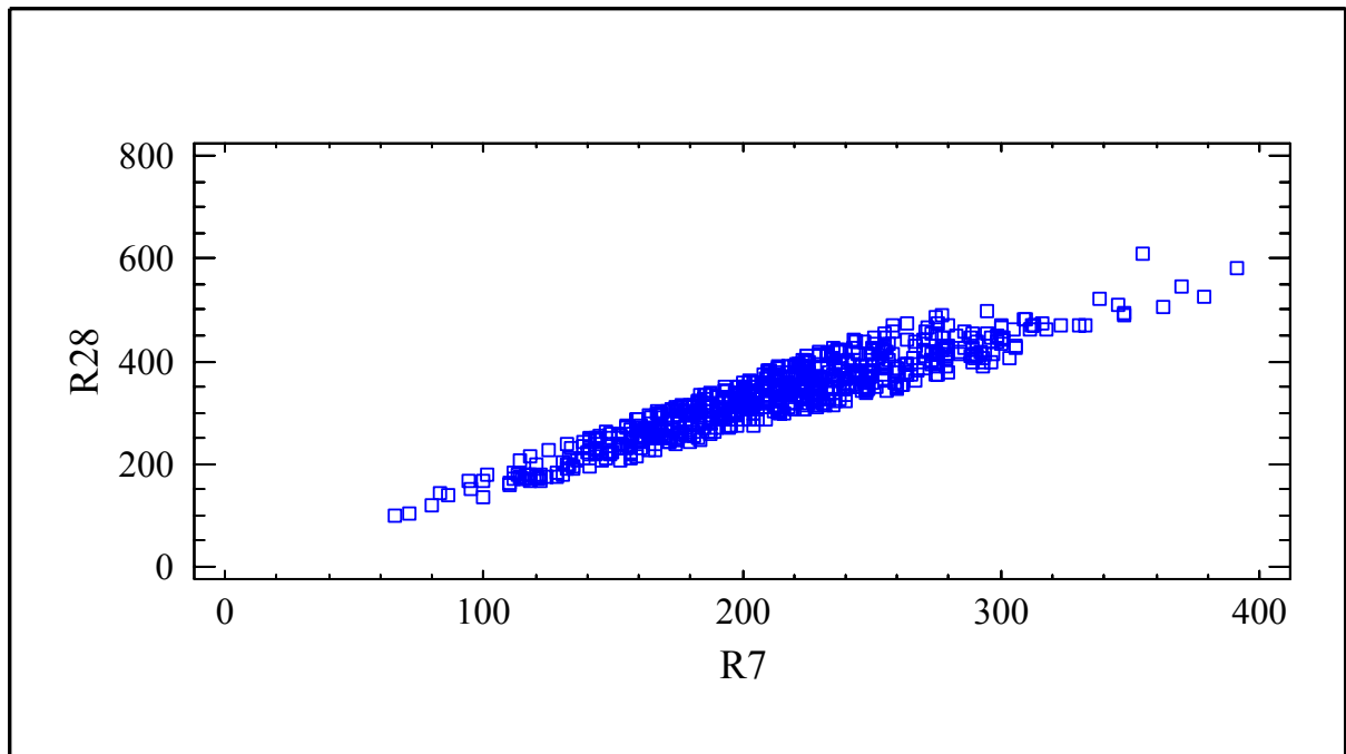
Gráfico 25.- Diagrama de Dispersión de R_{28} v/s R_7 ( \text{Kg}/\text{cm}^2 )
