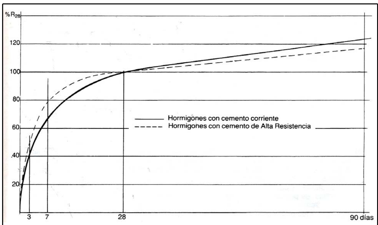
Gráfico 1.- Desarrollo de la resistencia en el tiempo, expresada como porcentaje de la resistencia a los 28 días
