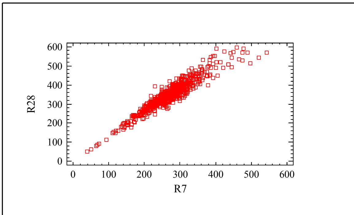
Gráfico 15.- Diagrama de Dispersión R_{28} v/s R_7 ( Kg/cm 2 )
