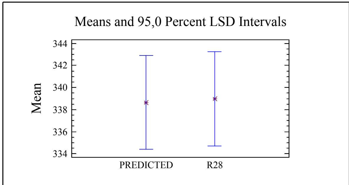
Gráfico 39.- Diferencia en la media de la variable observada y la predecida por fórmula elaborada para hormigones confeccionados con cementos corrientes.
