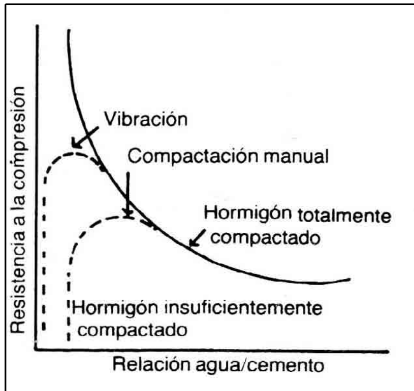
Figura 3.- Correspondencia entre la resistencia y la relación agua / cemento del hormigón.
