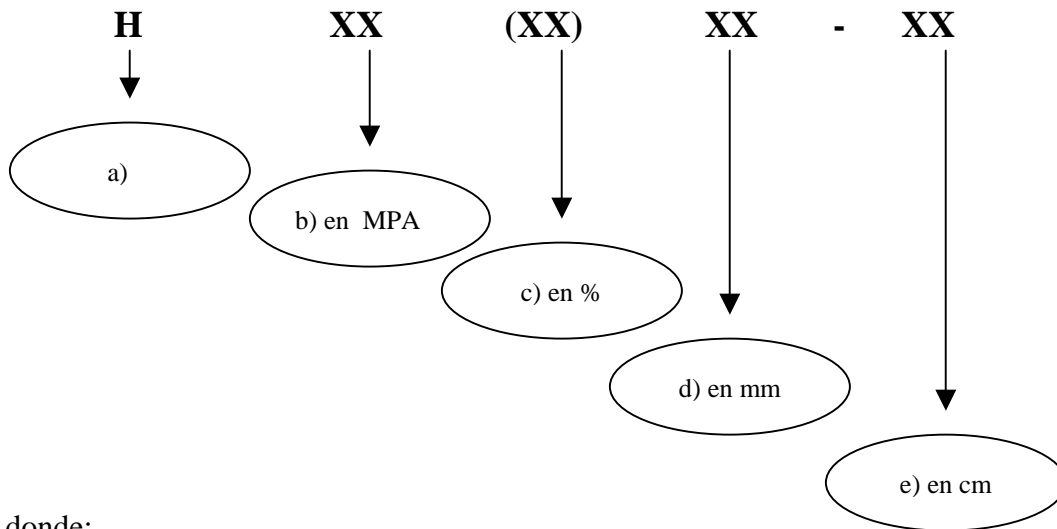
Figura 1.- Especificación en el nombre del hormigón según requerimientos.
