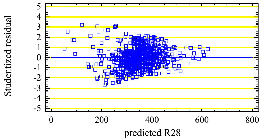
Gráfico 22.- Residual Plot
