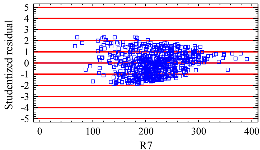
Gráfico 31.- Residual Plot
