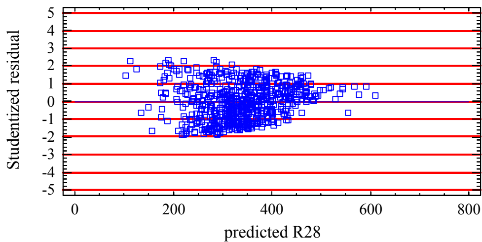
Gráfico 32.- Residual Plot
