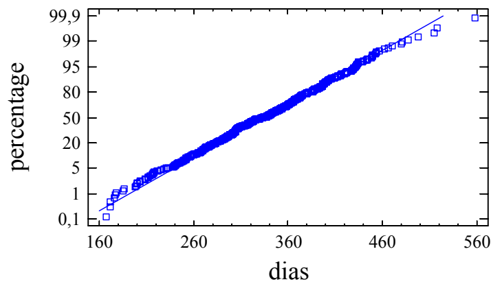
Gráfico 3.- Normal Probability Plot
